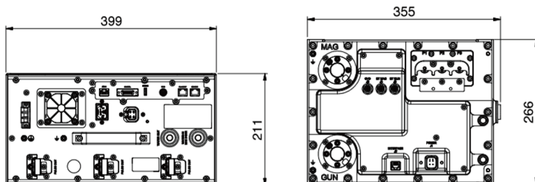
M110-i 寸法図
